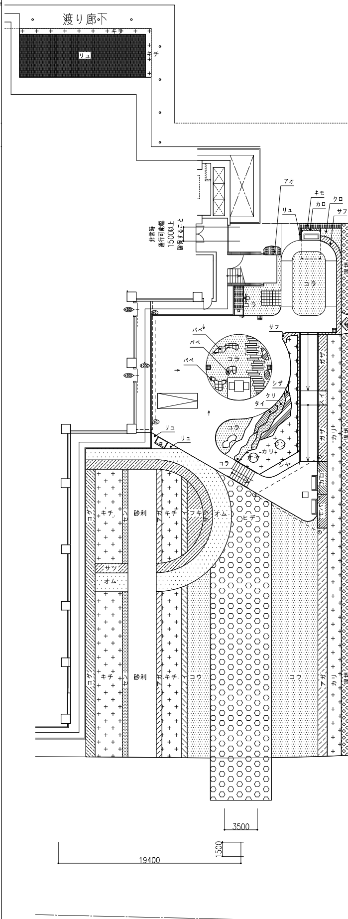
B1F サンクンガーデン 植栽計画図 S=1/100
