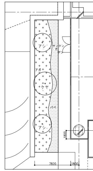
B1F サンクンガーデン 植栽計画図 S=1/100
